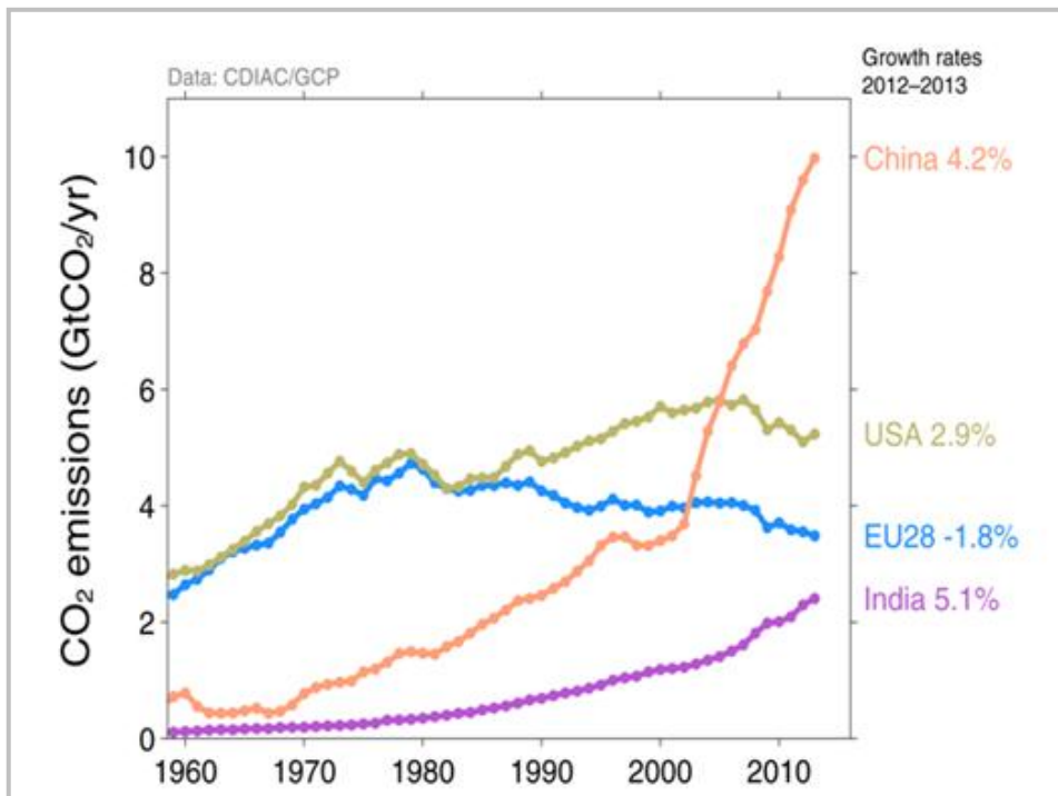
Figura 2. Di chi sono le responsabilità attuali delle emissioni carboniche
