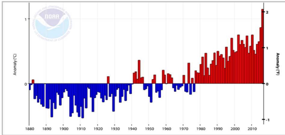
Figura 1. La crescita della temperatura media terrestre
