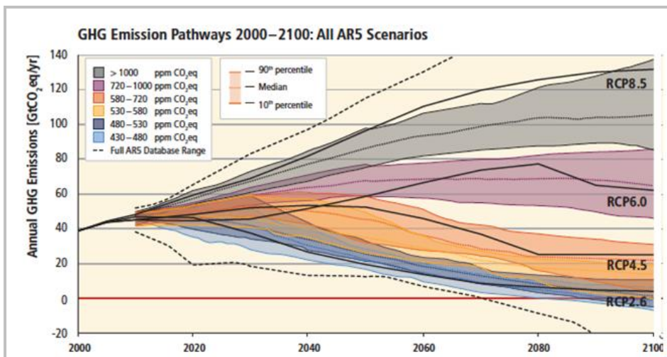
Figura 5. Gli scenari di questo secolo calcolati dal IPCC. Il RCP 2.6 è l'unico coerente con gli obiettivi di Parigi
