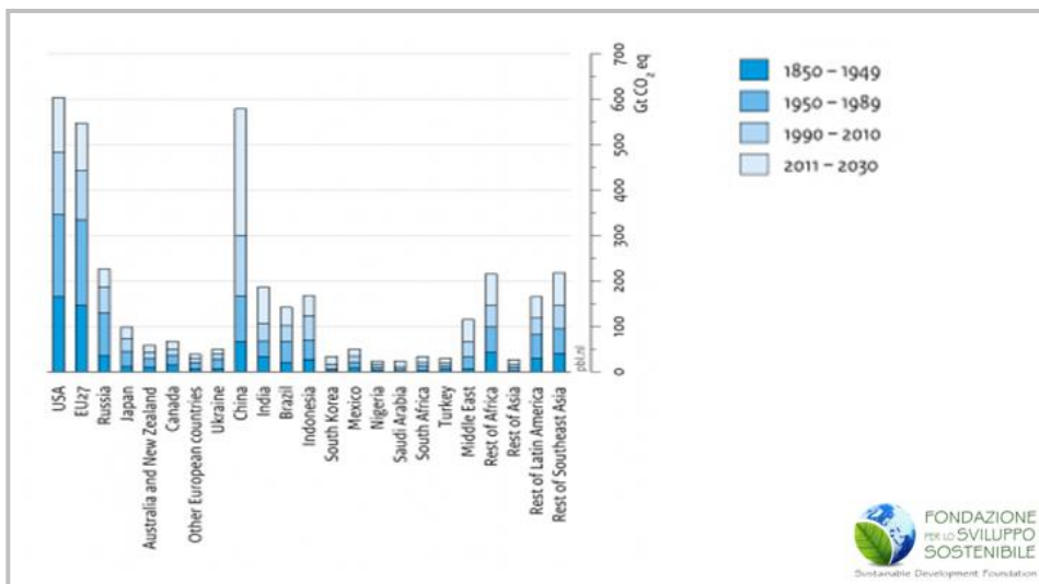
Figura 3. Di chi sono le responsabilità storiche delle emissioni carboniche e quindi del riscaldamento terrestre
