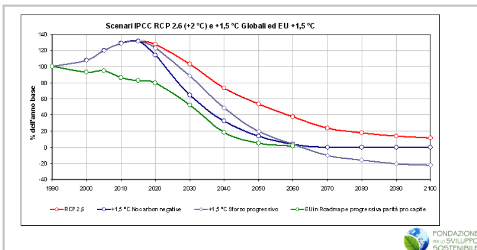
Figura 6. Gli scenari di questo secolo calcolati dalla Fondazione alla ipotesi del contenimento del riscaldamento globale a fine secolo entro 1,5 °C e del conseguente dimezzamento del Carbon Budget
