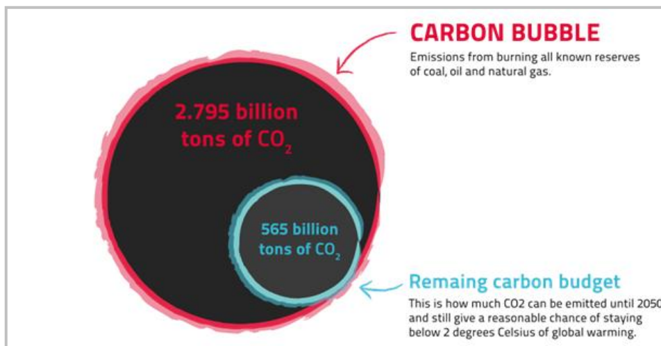
Figura 4. Il Carbon Budget: le emissioni cumulative massime residue
